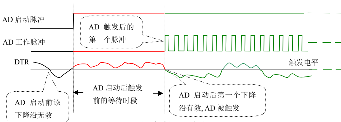
图 7.2 下降沿触发图例,上升沿同理
